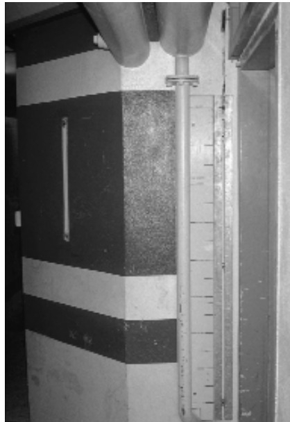
Von links nach rechts und von oben nach unten: Innenansichten des Artilleriewerks: Beobachtungsposten, Geschütz-Kasematte (leer), Telefonzentrale, Trinkwasser-Auffang- becken Unten: Getarnter Werkseingang
